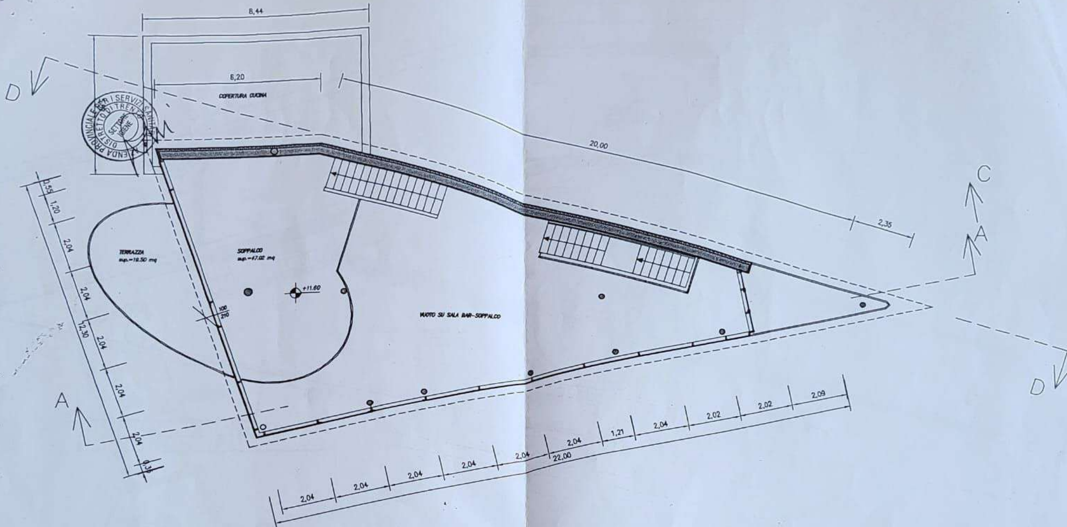
PIANTA SOPPALCO
